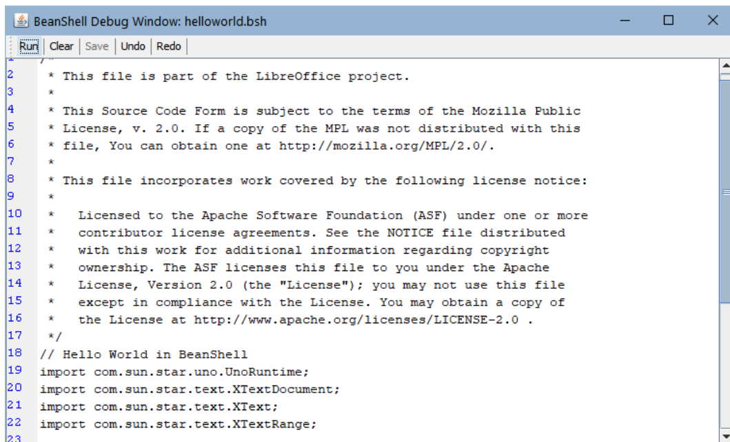
Figura 24: Ventana de depuración BeanShell
