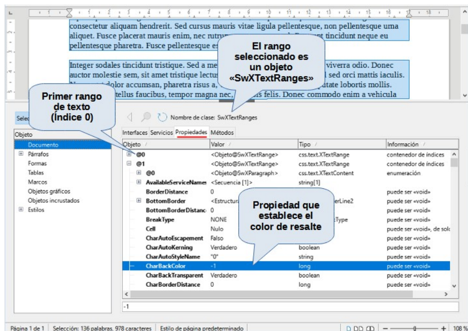
Figura 20: Uso del Inspector de objetos para buscar una propiedad
