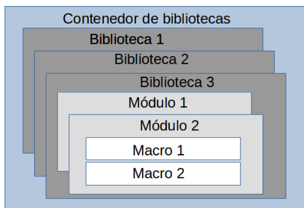
Figura 12: Jerarquía de las bibliotecas de macros
