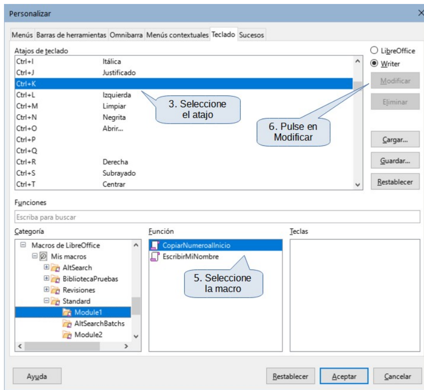
Figura 11: Asignar un atajo de teclado a una macro
