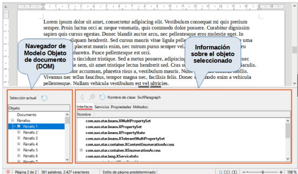
Figura 19: El Inspector de objetos UNO en un documento de Writer
