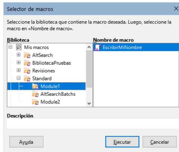
Figura 7: Diálogo Selector de macros
