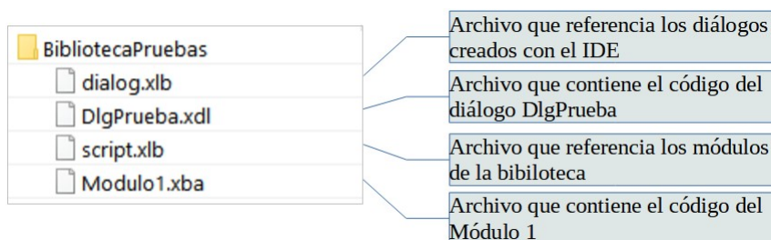
Figura 13: Contenido de la carpeta de la biblioteca exportada
