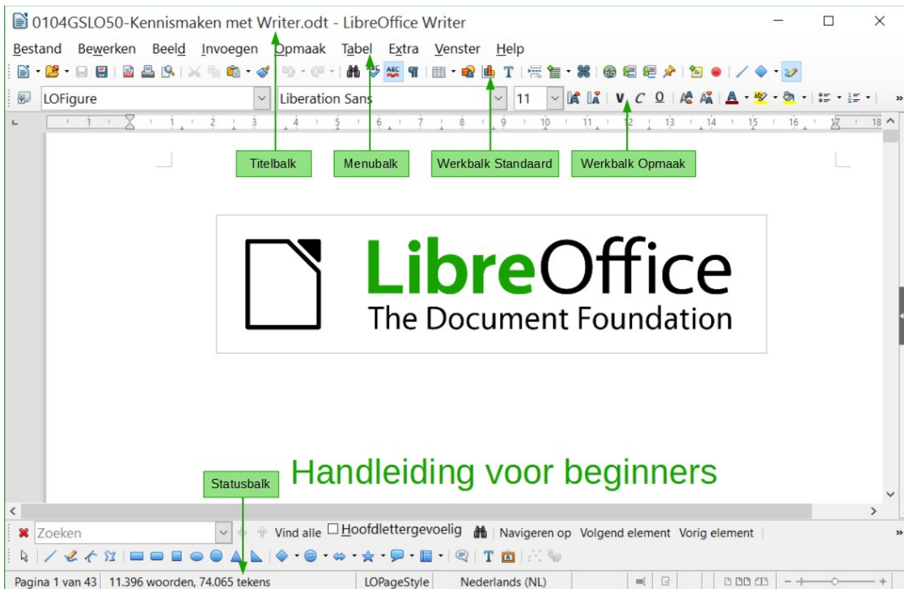
Afbeelding 1: De werkruimte van Writer in Afdruk-layout
