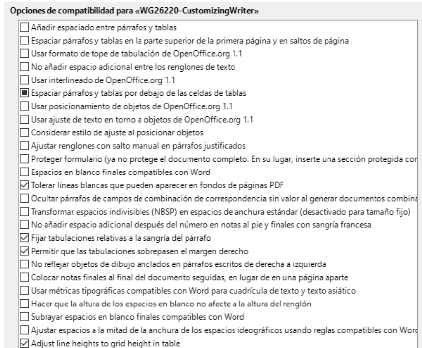
Figura 16: Opciones de Compatibilidad
