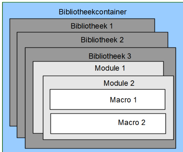
Afbeelding 7: hiërarchie Macrobibliotheek
