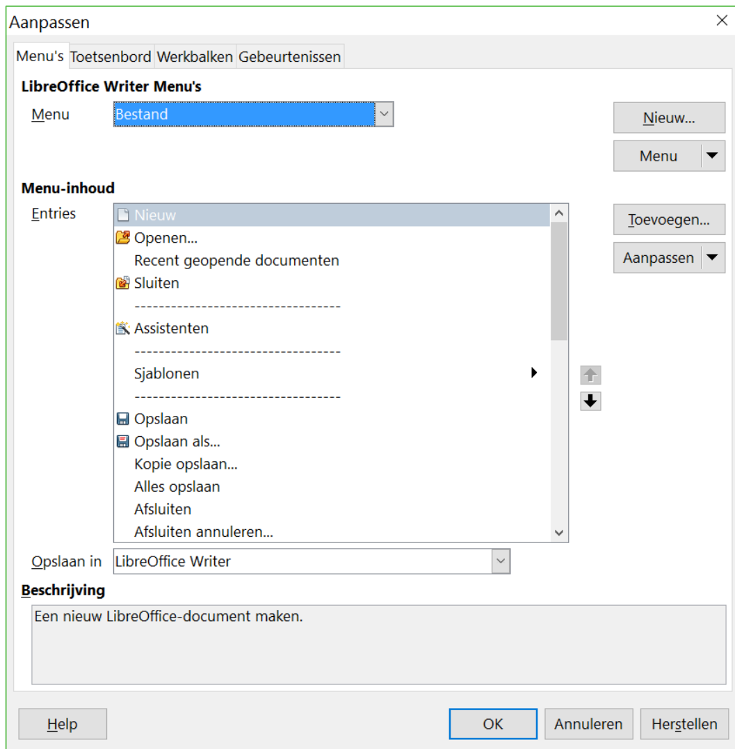
Afbeelding 10: dialoogvenster Aanpassen
