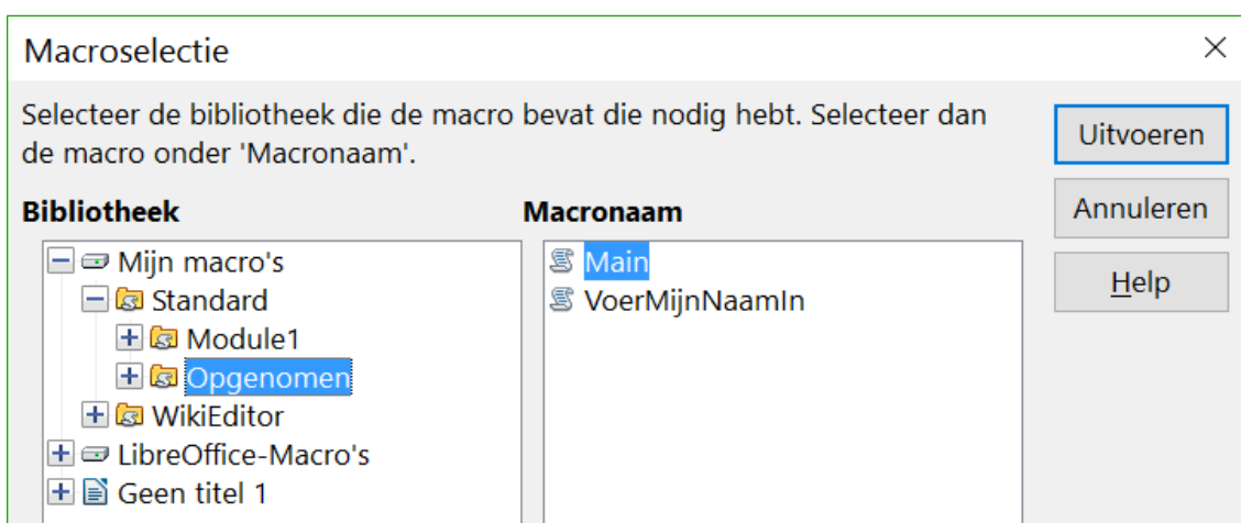
Afbeelding 5: Dialoogvenster Macroselectie
